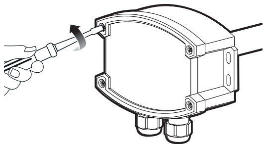
Рис. 3.d Открутите 4 винта
