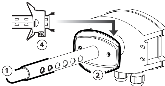
Рис. 3.e 1. Желательно выбрать подходящий участок воздуховода. Кончик датчика должен располагаться в хорошо проветриваемом месте. 2. Установите изолирующую площадку на воздуховод и закрепите ее 2 саморезами в соответствующих пазах. 3. Вставьте стержень датчика в изолирующий кронштейн. 4. Затяните винт кронштейна, чтобы зафиксировать датчик на воздуховоде.
